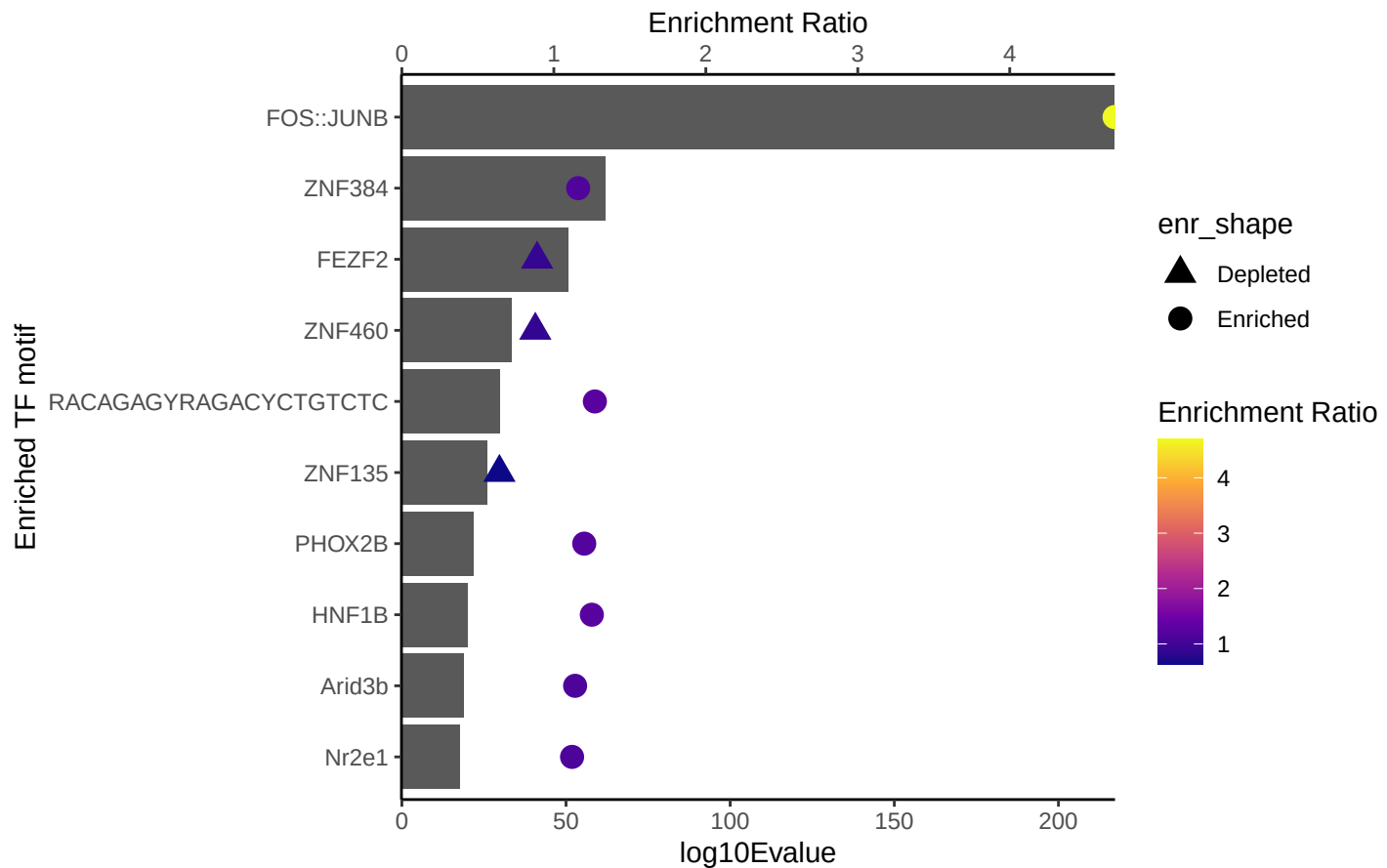
H3K27ac_Set2_data - 10
